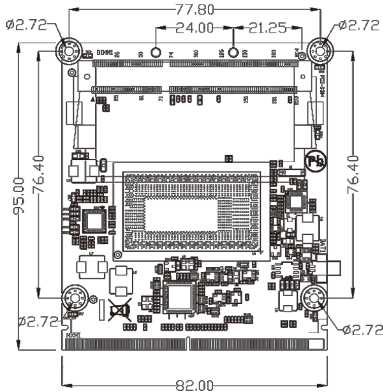
产品尺寸图(Unit:mm)
